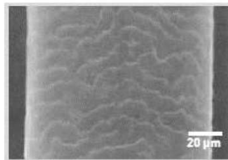
Cheveu déshydraté
